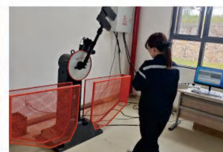
Pendulum impact testing machine 摆式冲击试验机
